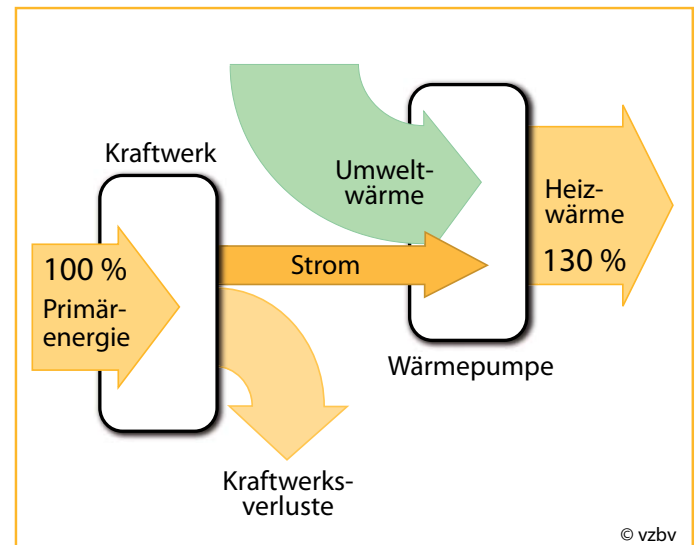
Energiebilanz einer Wärmepumpe mit Jahresarbeitszahl vier
